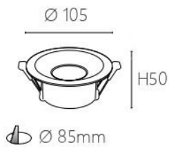
JBR 20803 材質：鋁材 尺寸：Ø105 H50 mm 嵌入孔：Ø85 mm (可適用 MR16)
