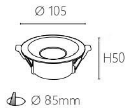
JBR 20804 材質：鋁材 尺寸：Ø105 H50 mm 嵌入孔：Ø85 mm (可適用 MR16)
