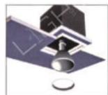
8. 燈下前環裝入光源
