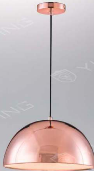
GLM-13758 3800 W300mm H170mm 線長1000mm E27 LEDx1 另計 銅材電鍍
