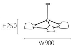
OK 20501 55000 W900 H250mm 線長1000mm E27 x 3另計 鋼材烤漆
