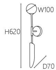
OK 20172 28000 W100 H620 D120mm G9 x 2另計 鋼材
