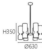
OK 20452 126000 Ø630 H350mm 桿長800mm E14 x 12另計 鋼材電鍍 玻璃 桿長400+400mm
