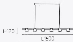
OK 20641 78000 L1500 H120mm 線長1500mm 內附LED 5Wx6 3000K 鋼材 玻璃
