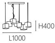
OK 20551 120000 L1000 W360 H400mm 線長1500mm 附LED 8W x 7 3000K 鋼材
