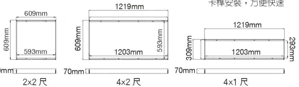
卡榫安裝，方便快捷
