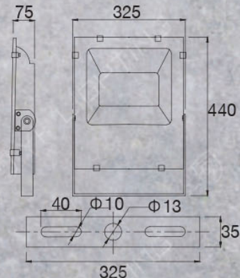
150W (單位: mm)
