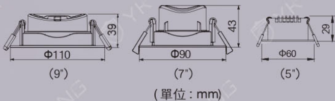
浩克氣氛光重點照明
