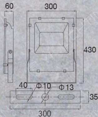
100W (單位: mm)
