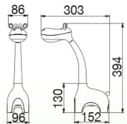
LED-DLGF6-Y (單位：mm)
