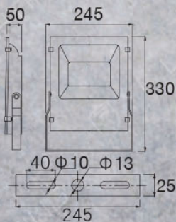
50W (單位: mm)
