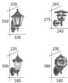
F3-20531 7600 W:320mm H:550mm D:330mm E27 LED 燈泡 X 1 另計 鋁製品烤漆 玻璃
